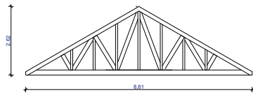
Szeglemezes (Gang Nail) rendszerű fa rúcsostartó gyártó által tervezve és készítve
