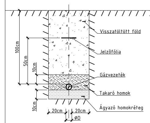
Munkaárok minta keresztmetsvény M=1:25
