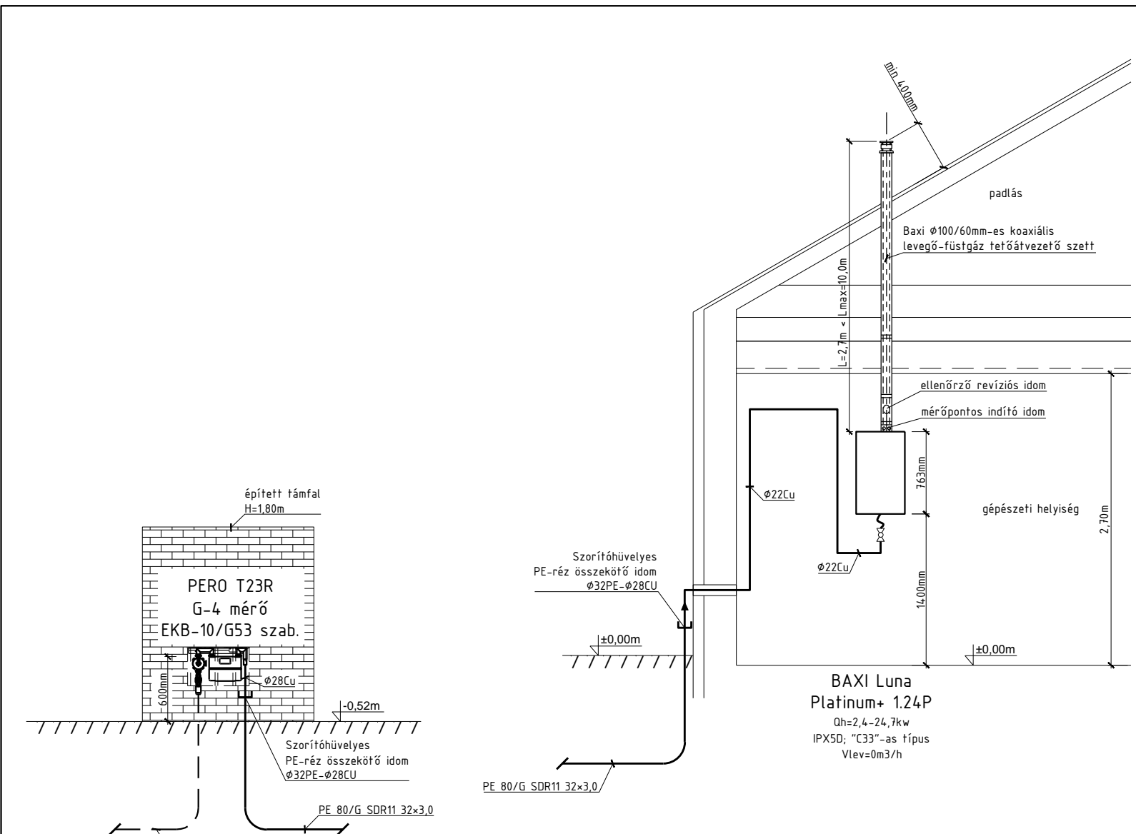
FÜGGŐLEGES CSŐTERV
