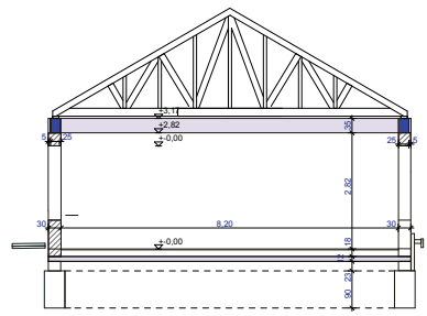
B-B metszet
