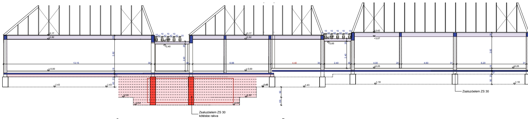
A-A metszet
