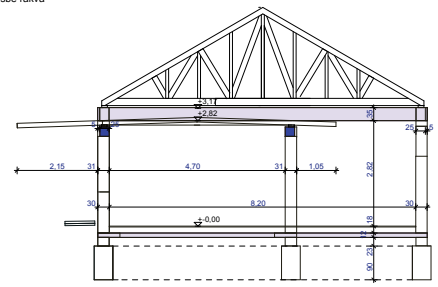
C-C metszet
